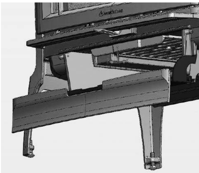
FIG. 5 - Tige de manœuvre de la grille
