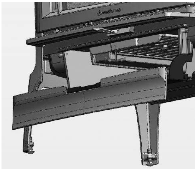
FIG. 5 - Mando agitador Parrilla
